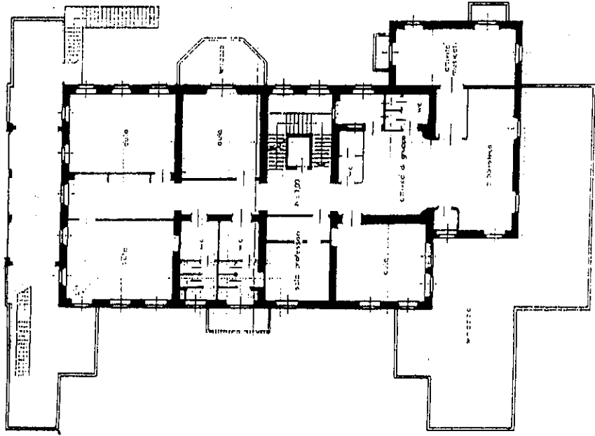
PIANO PRIMO
